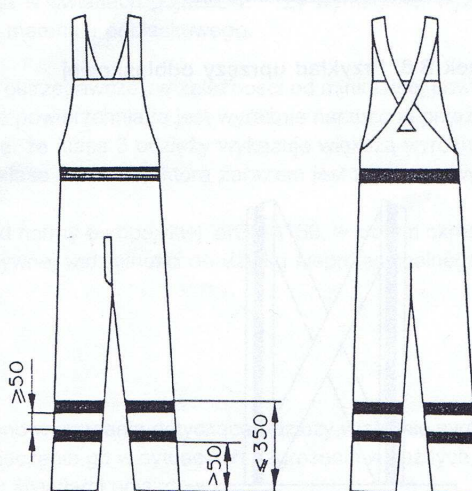
Rysunek B.6: Przykład spodni z podwyższonym przodem
