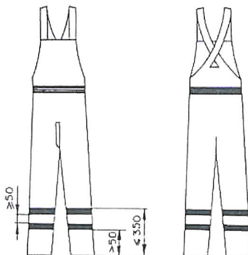
Rysunek B.6: Przykład spodni z podwyższonym przodem
