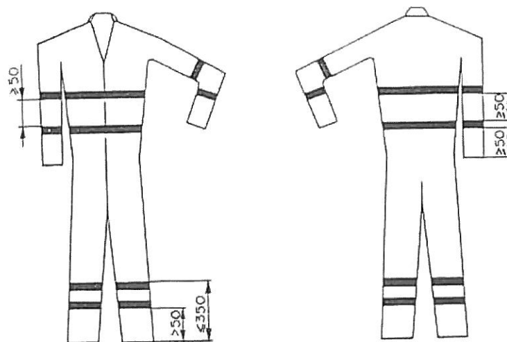
Rysunek B.1: Przykład kombinezonu
