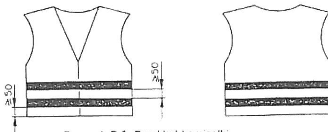
Rysunek B.3: Przykład kamizelki
