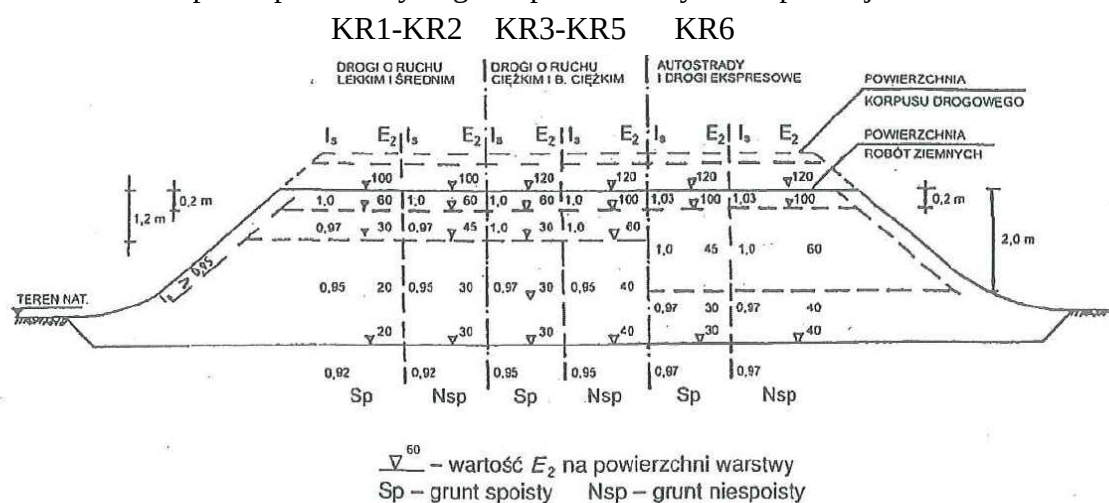
Rysunek 1. Minimalne wartości wskaźnika zagęszczenia gruntu w nasypach
